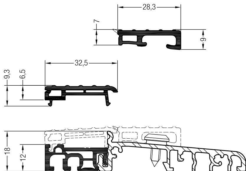
Set Bodenschwelle außenöffnend Bautiefe 86
