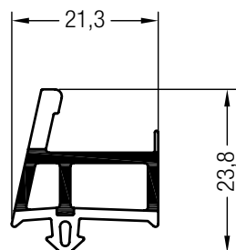
Passivhaus-Mittelsteg
