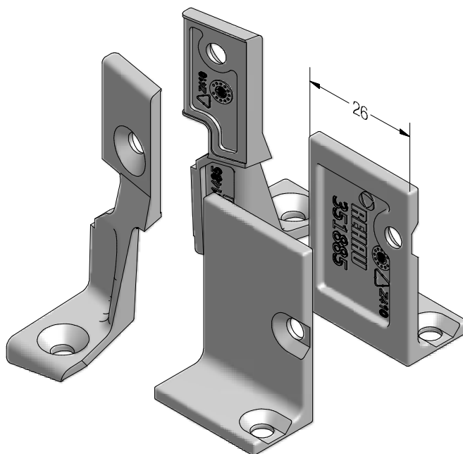
Set Pfostenwinkel GENE0®
