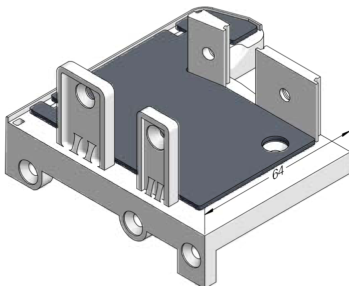
Schwellenhalter Blendrahmen 90
