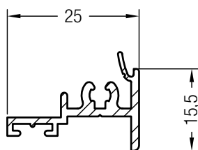
Deckleiste Flügel T GENE0®
