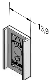
Abdeckkappe Schwellenhalter GENEORASA
