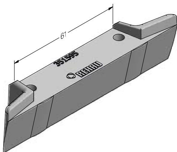
Dichtblock Pfosten 126 GENE0®
