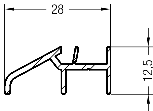
Wetterschenkel 12,5 GENEORASA
