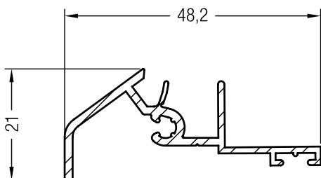
Wetterschenkel 21 GENEORASA
