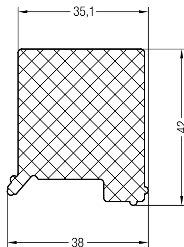
TM 35 x 42
