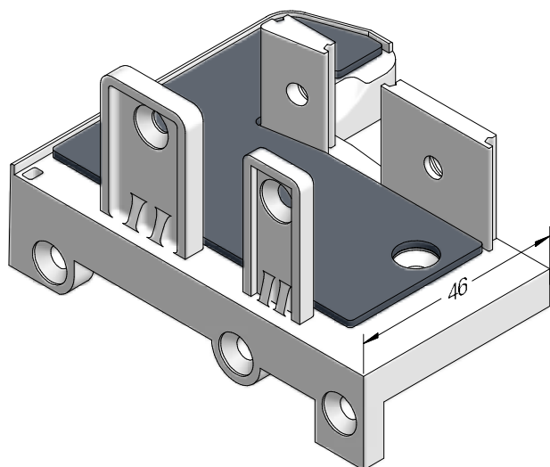
Schwellenhalter Blendrahmen 72
