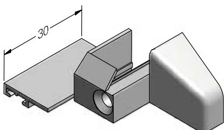
Endkappe Wetterschenkel 21 GENE0®
