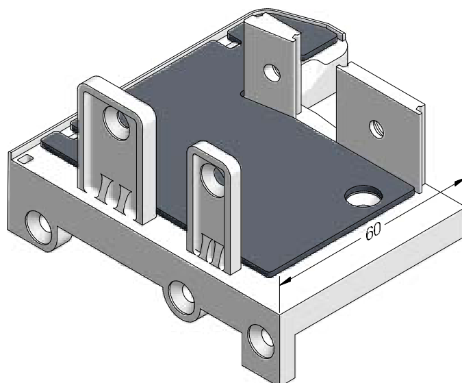
Schwellenhalter Blendrahmen 86 GENE0®
