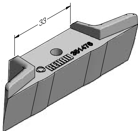
Dichtblock Pfosten 98 GENE0®
