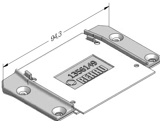
Mechanischer Verbinder Pfosten 112 ED 86 plus/HT Flügel T GENE0® Zink-Druckguss
