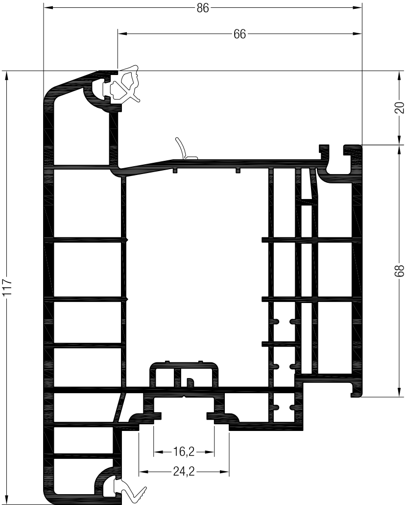
Flügel
