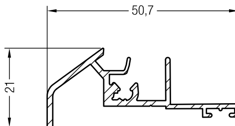
Wetterschenkel Haustür GENEORAPHZ
