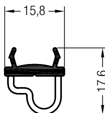
Kältestopp
