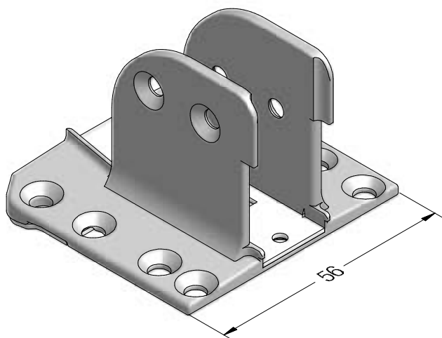
Mechanischer Verbinder Sprosse 64/86 Zink-Druckguss
