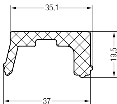
TM 35 x 20
