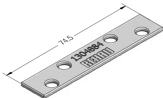
Montageplatte Pfosten 98 und 126 GENE0® (in Verbindung mit Blendrahmen 72 und 90) Stahl verzinkt
