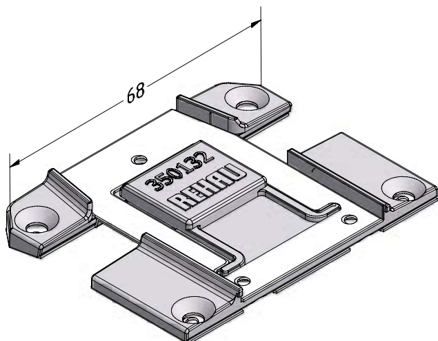
Mechanischer Verbinder Pfosten 98 GENE0®
