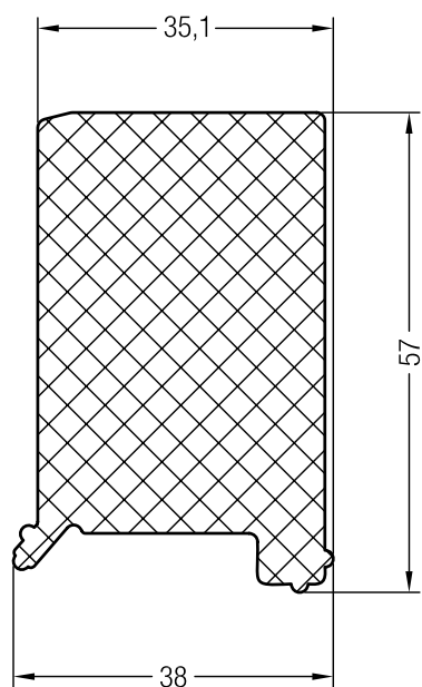
TM 35 x 57
